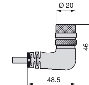
Bild 8-13: Steckverbinder BKS-S233-PU-__
