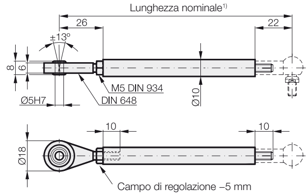
Fig. 8-4: Asta di comando BTL2-GS10-____-A
