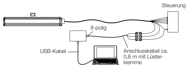
Bild 6-2: Anschluss der Kommunikationsbox mit Kabelanschluss
