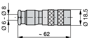
Fig. 8-10 : Connecteur BKS-S32M-00
