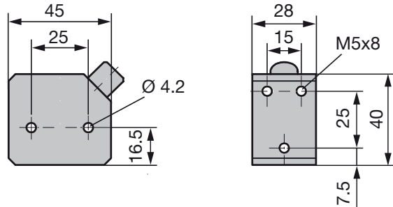
Fig. 8-9: Medidas de montaje del sensor de posición BTL5-P-4500-1
