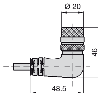
Fig. 8-13 : Connecteur BKS-S233-PU-__
