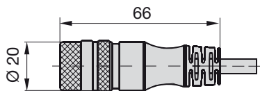
Fig. 8-12 : Connecteur BKS-S232-PU-__
