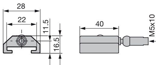
Fig. 8-3: Medidas de montaje del sensor de posición BTL5-T-2814-1S
