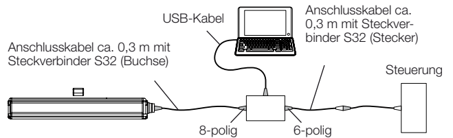
Bild 6-1: Anschluss der Kommunikationsbox mit Steckverbinder
