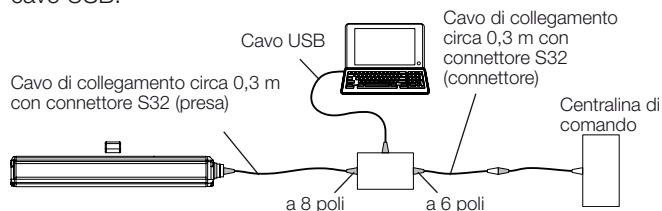
Fig. 6-1: Collegamento della scatola di comunicazione con connettore
