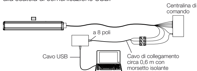
Fig. 6-2: Collegamento della scatola di comunicazione con cavo
