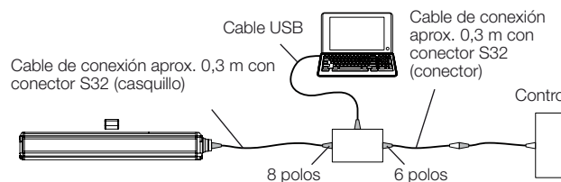
Fig. 6-1: Conexión del módulo de comunicación con conector
