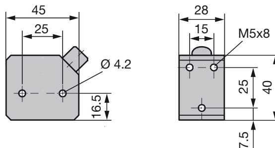
Fig. 8-9: Dimensioni di ingombro datore di posizione BTL5-P-4500-1
