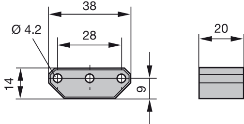
Fig. 8-5: Medidas de montaje del sensor de posición BTL5-P-3800-2
