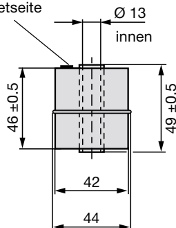
Bild 1: Abmessungen des Schwimmers BTL2-S-4414-4Z
