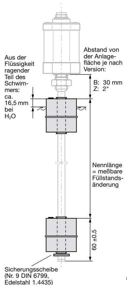
Bild 3: Füllstandsmessung mit Schwimmer BTL2-S-4414-4Z und Wegaufnehmer-Version BTL...B/Z...
