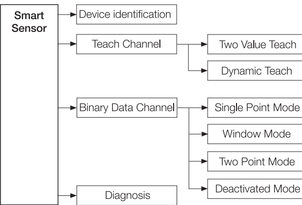
Bild 4: Funktionen des Smart Sensors
