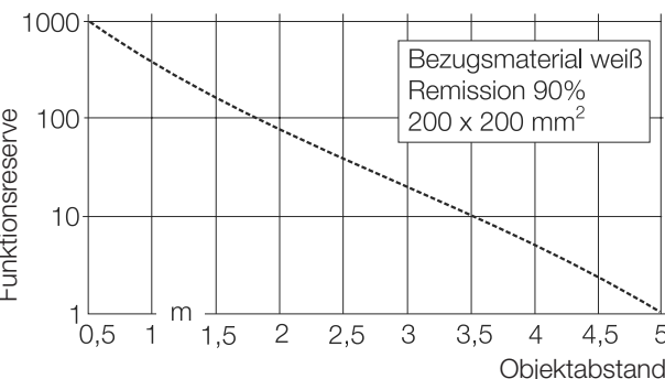
Bild 3: Funktionsreserve in Abhängigkeit vom Objektstand
