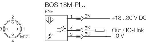
Bild 2: Anschluss-Schaltbild, Steckerbild
