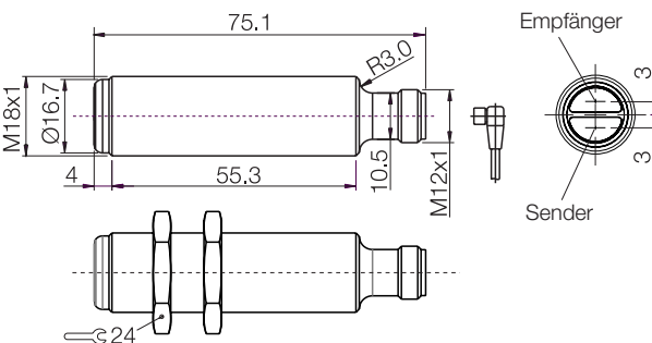
Bild 1: Abmessungen
