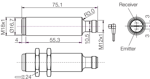
Fig. 1: Dimensions
