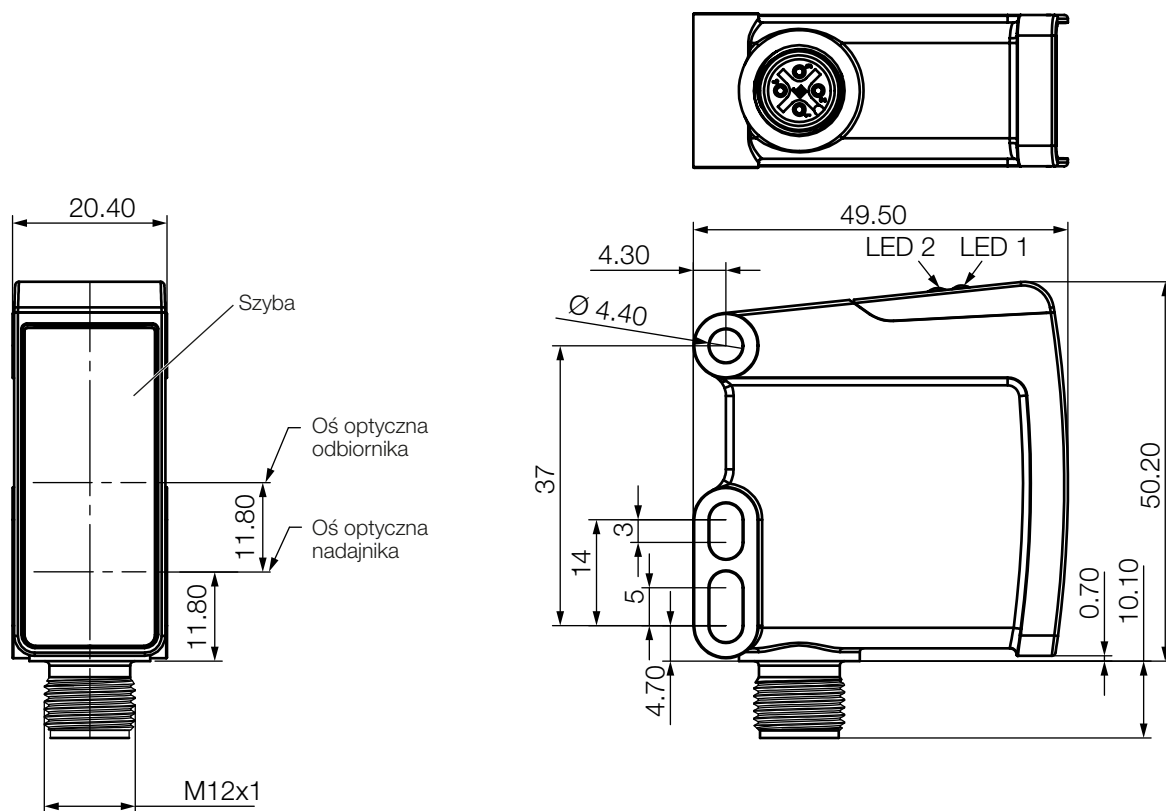
Rys. 4-1: Wymiary, budowa i działanie
