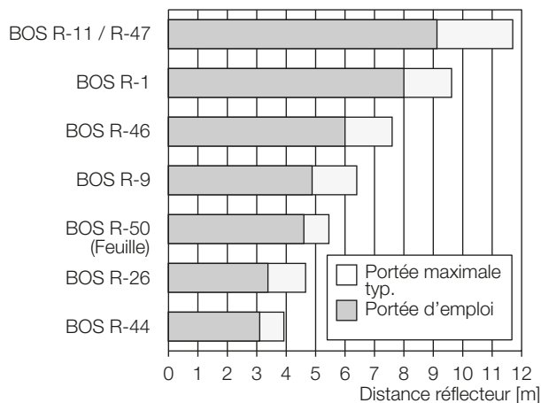
Fig. 9-1 : Portées
