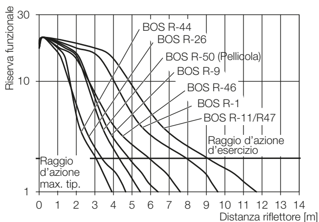
Fig. 9-2: Riserva funzionale sulla distanza
