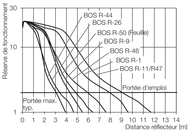
Fig. 9-2 : Réserve de fonctionnement sur la distance
