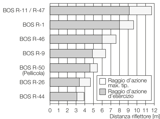
Fig. 9-1: Raggi d'azione
