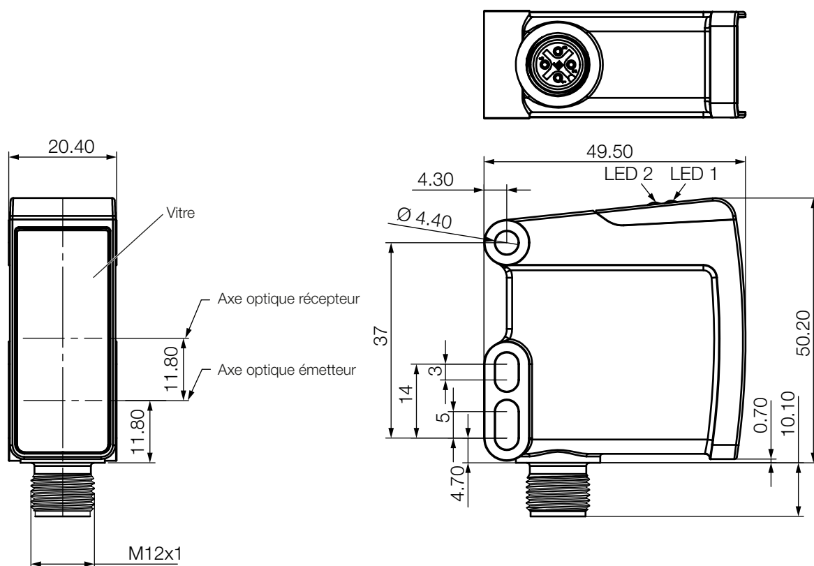
Fig. 4-1 : Dimensions, structure et fonction
