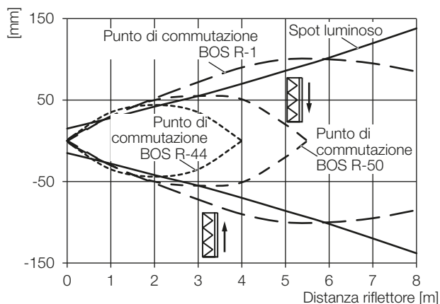
Fig. 9-3: Curva di avvio
