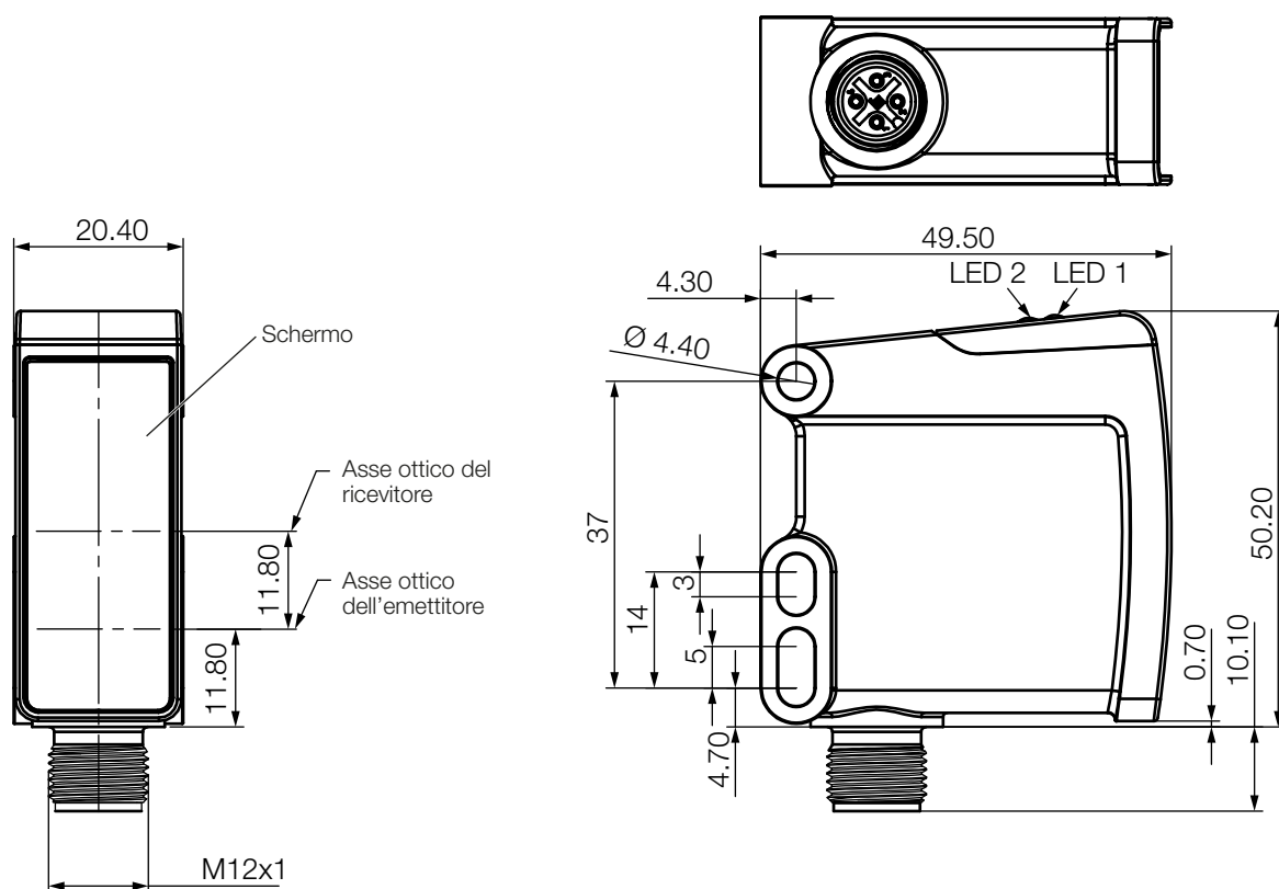
Fig. 4-1: Dimensioni, struttura e funzionamento
