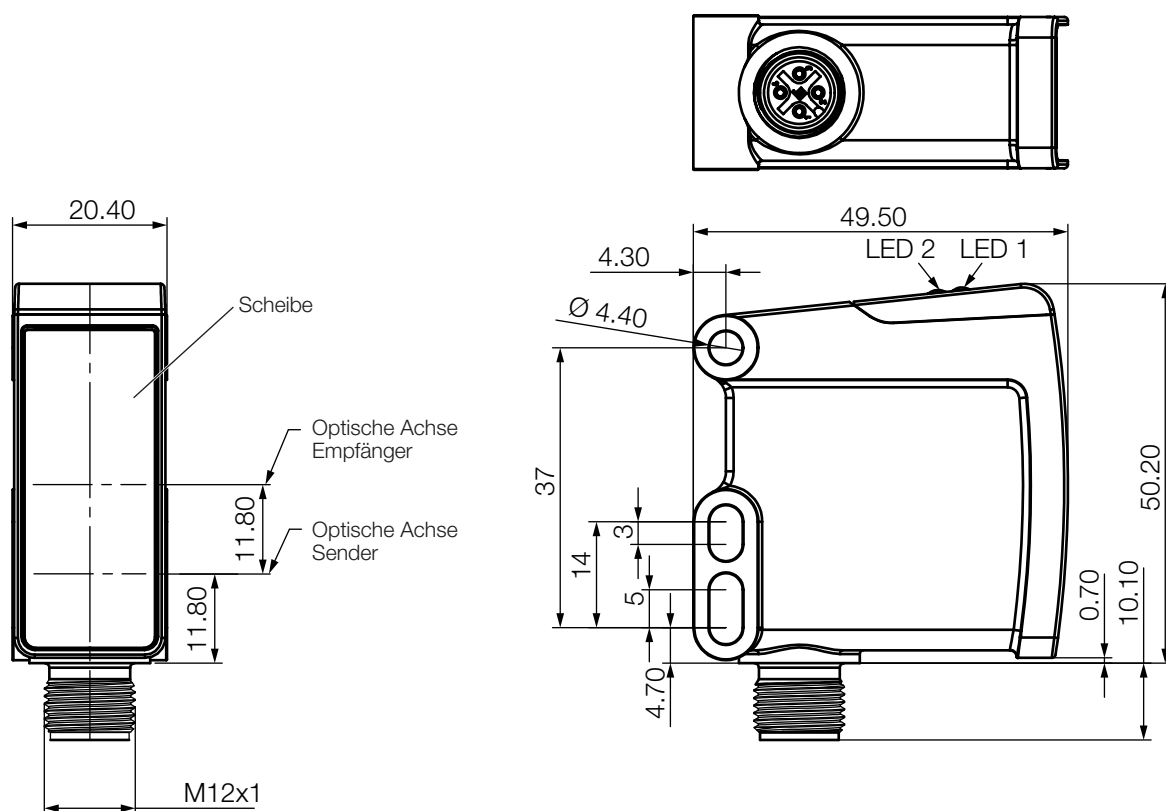
Bild 4-1: Abmessungen, Aufbau und Funktion
