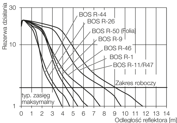
Rys. 9-2: Rezerwa działania na odległości
