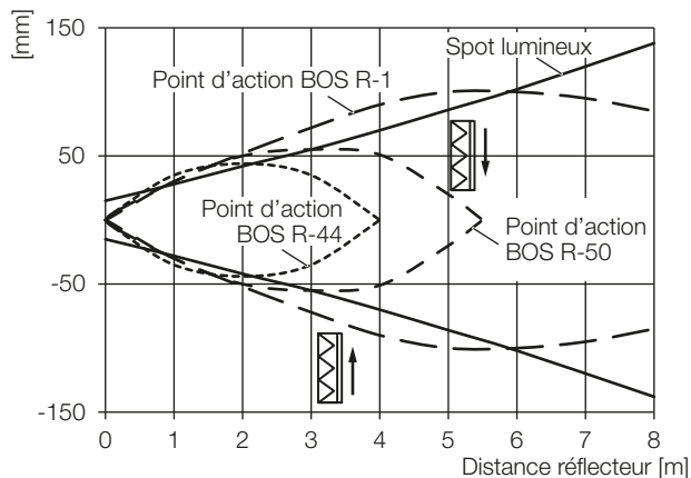
Fig. 9-3 : Courbe de détection
