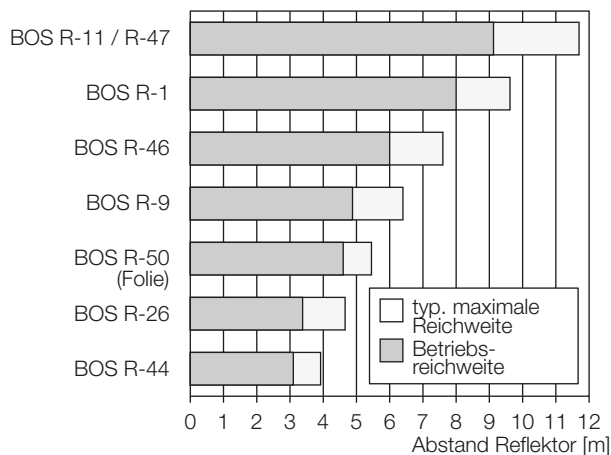
Bild 9-1: Reichweiten
