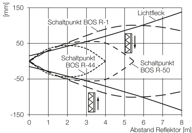
Bild 9-3: Anfahrkurve
