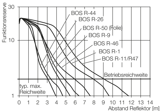
Bild 9-2: Funktionsreserve über den Abstand
