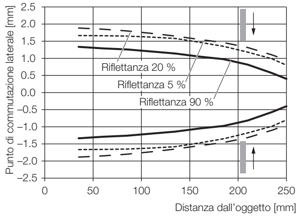
Fig. 9-4: Punto di commutazione laterale (...-LH10-...)
