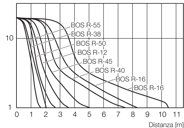
Fig. 9-15: Riserva funzionale sulla distanza (...-LK10-...)
