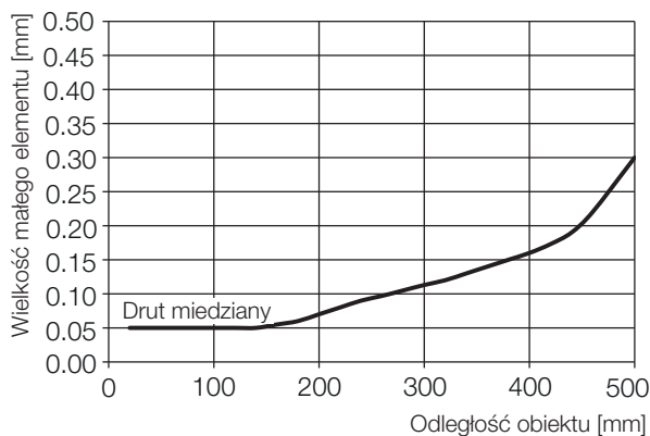
Rys. 9-11: Najmniejszy możliwy do wykrycia element (...-LH11-...)
