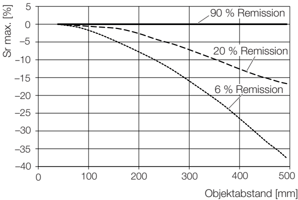
Bild 9-2: Schaltabstandsabweichung (...-LH11-...)
