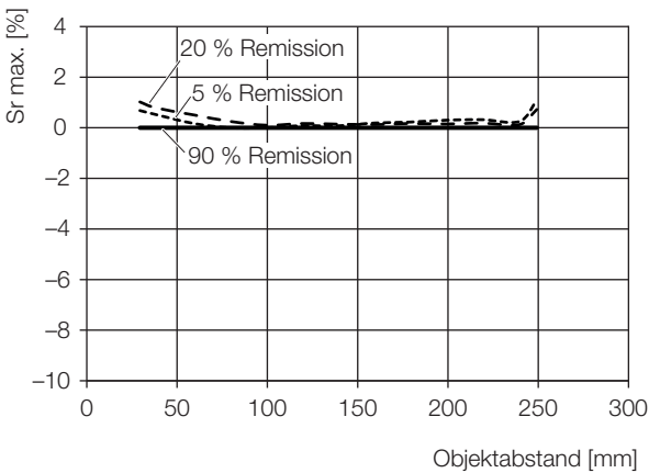
Bild 9-1: Schaltabstandsabweichung (...-LH10-...)
