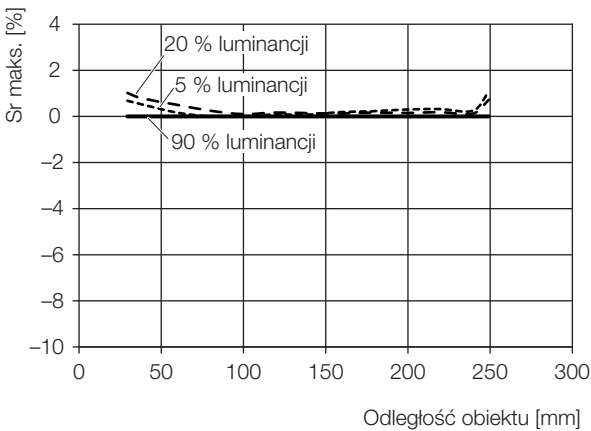
Rys. 9-1: Odchylenie odległości przełączania (...-LH10-...)
