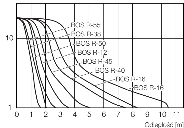
Rys. 9-15: Rezerwa działania na odległości (...-LK10-...)
