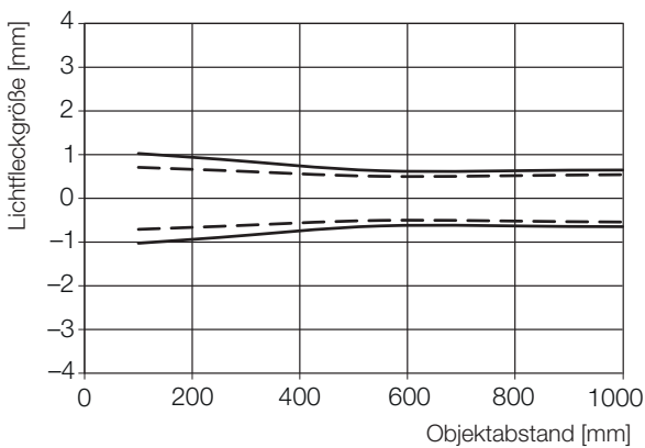
Bild 9-9: Lichtfleckgröße (...-LH12-...)
