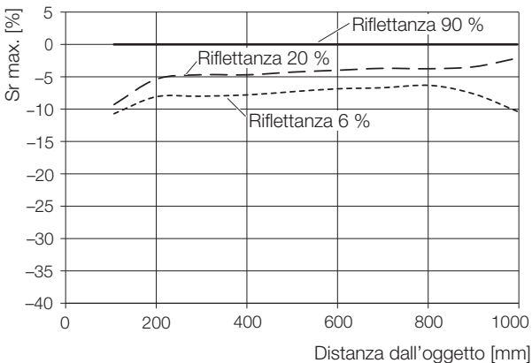
Fig. 9-3: Scostamento distanza di commutazione (...-LH12-...)
