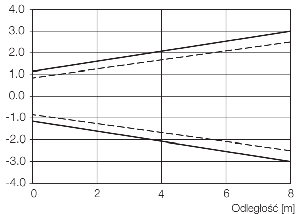
Rys. 9-14: Wielkość plamki światła (...-LK10-...)
