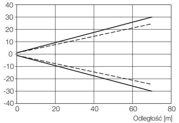
Rys. 9-16: Wielkość plamki światła (...-LS10-...)
