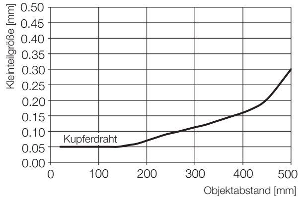
Bild 9-11: Kleinstes erkennbares Teil (...-LH11-...)
