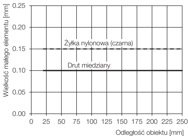
Rys. 9-10: Najmniejszy możliwy do wykrycia element (...-LH10-...)
