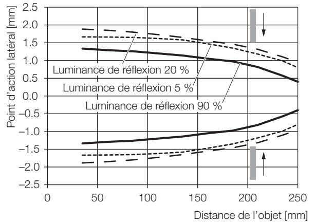
Fig. 9-4: Point d'action latéral (...-LH10-...)
