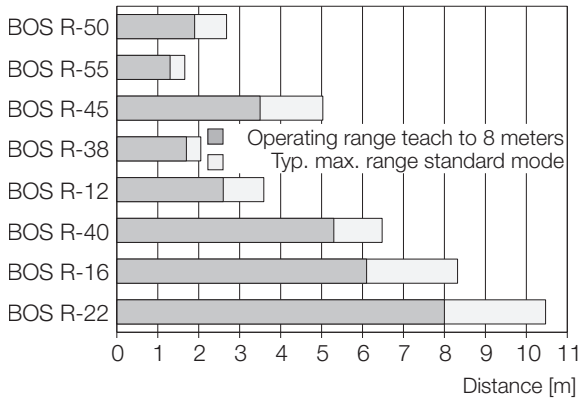
Fig. 9-13: Ranges (...-LK10-...)
