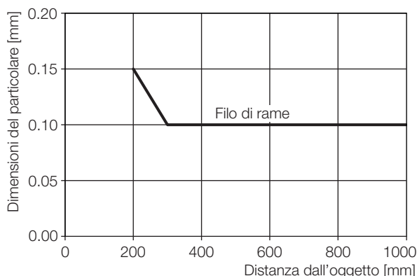
Fig. 9-12: Minimo particolare riconoscibile (...-LH12-...)
