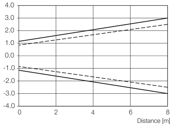
Fig. 9-14: Taille du spot lumineux (...-LK10-...)
