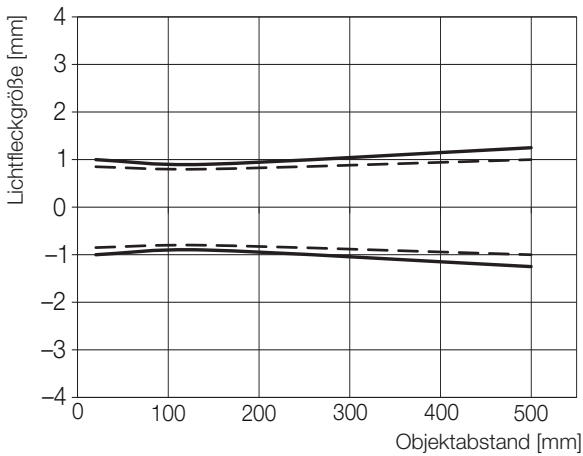
Bild 9-8: Lichtfleckgröße (...-LH11-...)
