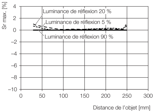
Fig. 9-1: Écart de portée (...-LH10-...)
