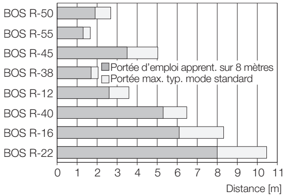
Fig. 9-13: Portées (...-LK10-...)
