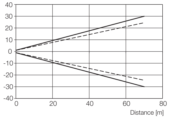
Fig. 9-16: Taille du spot lumineux (...-LS10-...)
