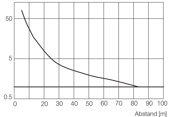
Bild 9-17: Funktionsreserve über den Abstand (...-LS10/LE10-...)
