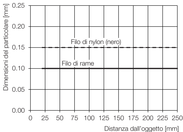
Fig. 9-10: Minimo particolare riconoscibile (...-LH10-...)
