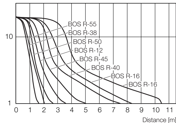
Fig. 9-15: Gain excédentaire sur la distance (...-LK10-...)
