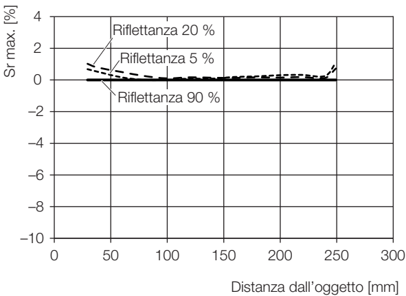
Fig. 9-1: Scostamento distanza di commutazione (...-LH10-...)
