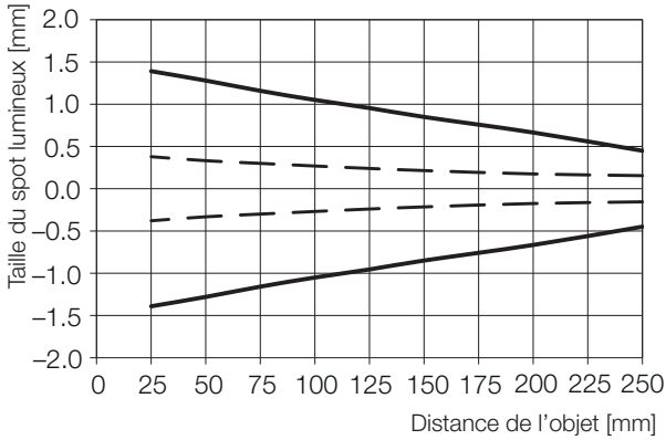
Fig. 9-7: Taille du spot lumineux (...-LH10-...)
