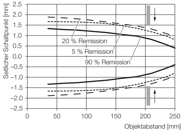
Bild 9-4: Seitlicher Schaltpunkt (...-LH10-...)
