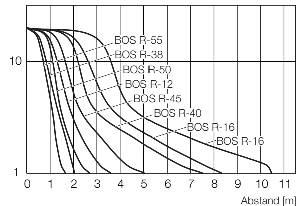
Bild 9-15: Funktionsreserve über den Abstand (...-LK10-...)
