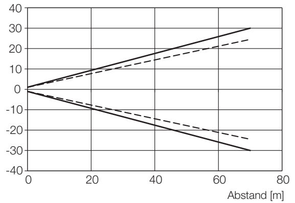
Bild 9-16: Lichtfleckgröße (...-LS10-...)
