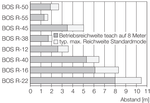
Bild 9-13: Reichweiten (...-LK10-...)
