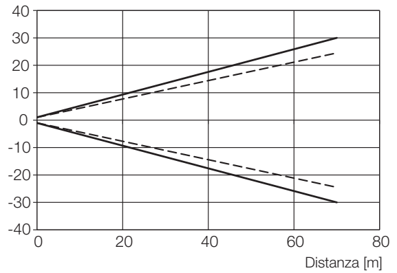
Fig. 9-16: Dimensioni dello spot luminoso (...-LS10-...)
