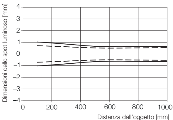
Fig. 9-9: Dimensioni dello spot luminoso (...-LH12-...)
