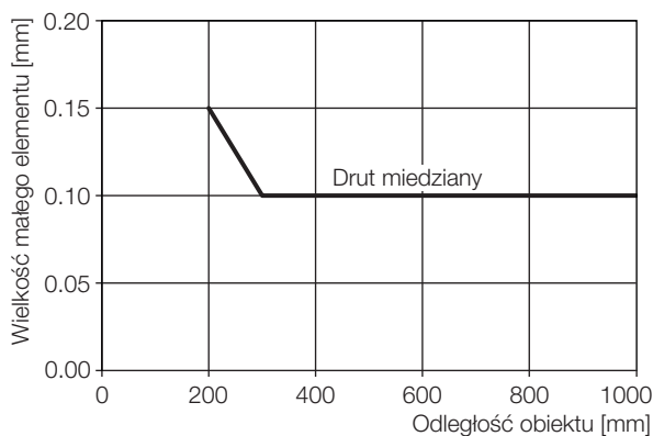
Rys. 9-12: Najmniejszy możliwy do wykrycia element (...-LH12-...)
