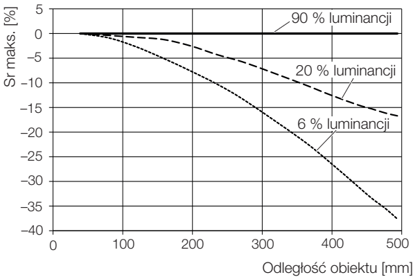
Rys. 9-2: Odchylenie odległości przełączania (...-LH11-...)
