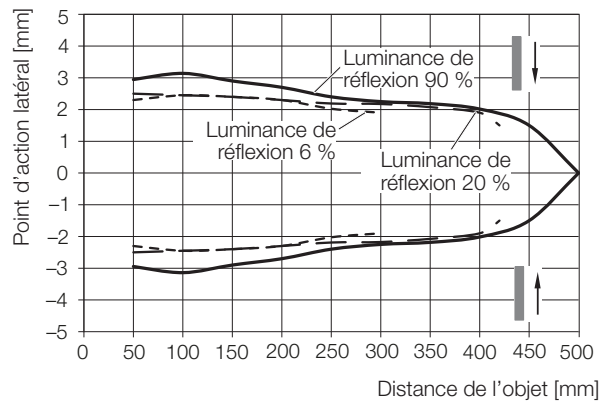
Fig. 9-5: Point d'action latéral (...-LH11-...)
