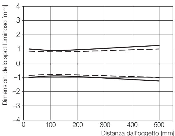
Fig. 9-8: Dimensioni dello spot luminoso (...-LH11-...)
