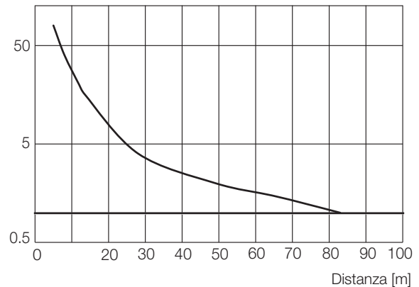
Fig. 9-17: Riserva funzionale sulla distanza (...-LS10/LE10-...)
