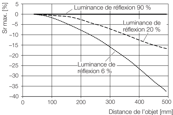
Fig. 9-2: Écart de portée (...-LH11-...)
