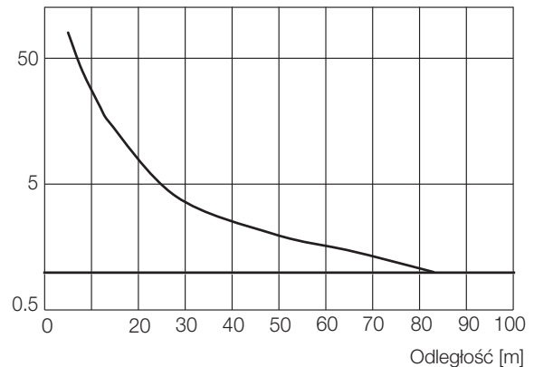
Rys. 9-17: Rezerwa działania na odległości (...-LS10/LE10-...)
