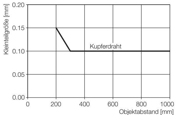
Bild 9-12: Kleinstes erkennbares Teil (...-LH12-...)
