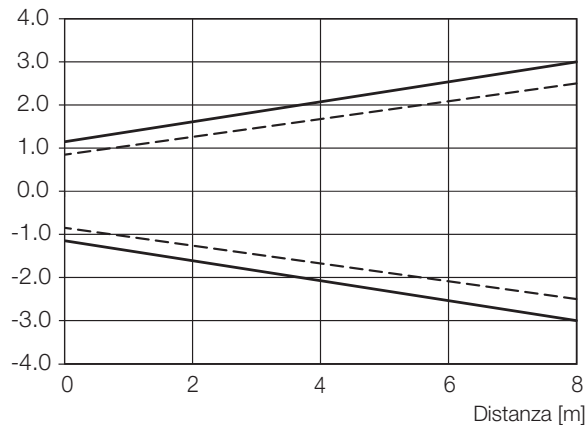
Fig. 9-14: Dimensioni dello spot luminoso (...-LK10-...)
