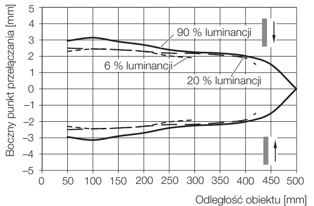
Rys. 9-5: Boczny punkt przełączania (...-LH11-...)
