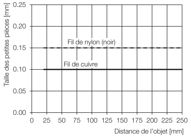
Fig. 9-10: Plus petite pièce reconnaissable (...-LH10-...)
