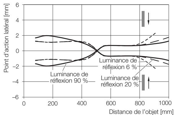
Fig. 9-6: Point d'action latéral (...-LH12-...)
