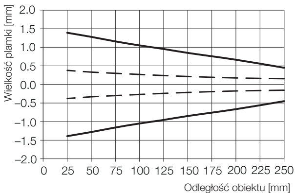
Rys. 9-7: Wielkość plamki światła (...-LH10-...)
