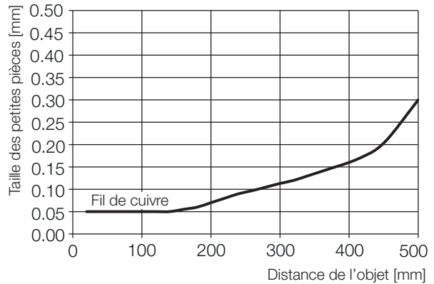
Fig. 9-11: Plus petite pièce reconnaissable (...-LH11-...)
