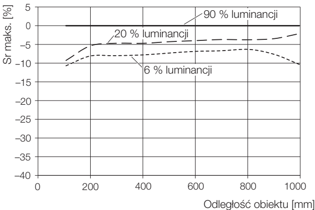
Rys. 9-3: Odchylenie odległości przełączania (...-LH12-...)
