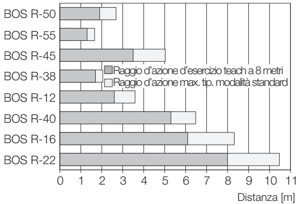
Fig. 9-13: Raggi d'azione (...-LK10-...)
