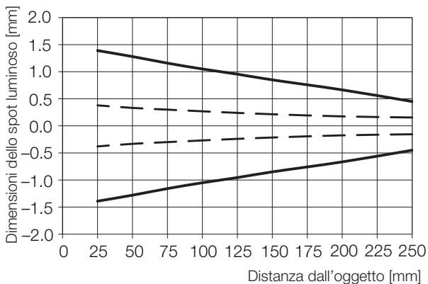
Fig. 9-7: Dimensioni dello spot luminoso (...-LH10-...)
