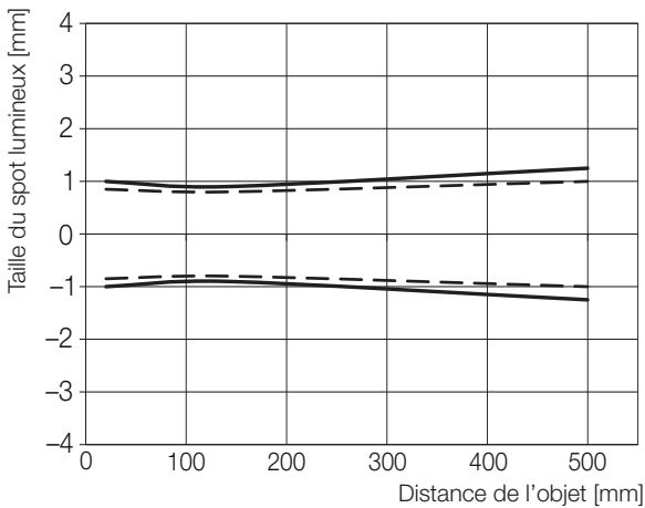
Fig. 9-8: Taille du spot lumineux (...-LH11-...)
