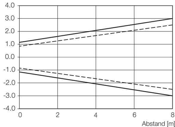
Bild 9-14: Lichtfleckgröße (...-LK10-...)
