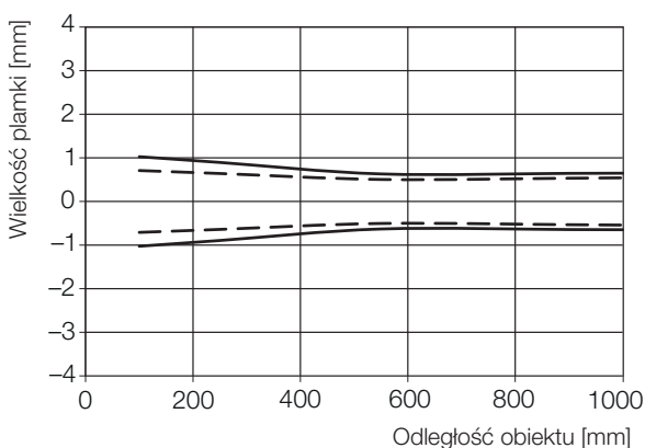
Rys. 9-9: Wielkość plamki światła (...-LH12-...)
