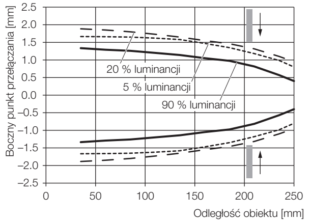
Rys. 9-4: Boczny punkt przełączania (...-LH10-...)
