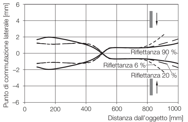
Fig. 9-6: Punto di commutazione laterale (...-LH12-...)
