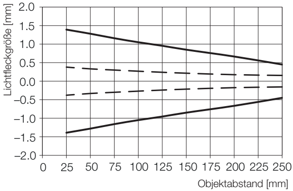
Bild 9-7: Lichtfleckgröße (...-LH10-...)
