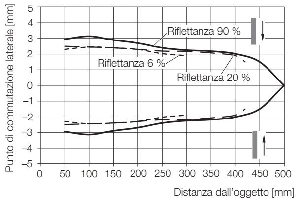
Fig. 9-5: Punto di commutazione laterale (...-LH11-...)
