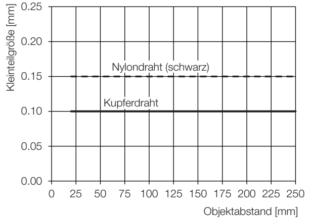
Bild 9-10: Kleinstes erkennbares Teil (...-LH10-...)
