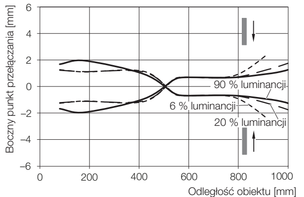
Rys. 9-6: Boczny punkt przełączania (...-LH12-...)
