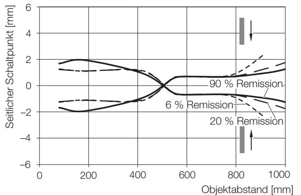
Bild 9-6: Seitlicher Schaltpunkt (...-LH12-...)
