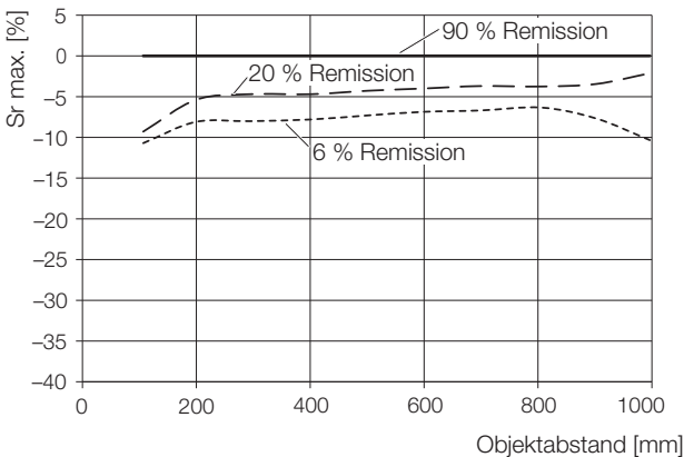
Bild 9-3: Schaltabstandsabweichung (...-LH12-...)
