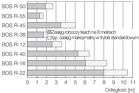
Rys. 9-13: Zasięg (...-LK10-...)
