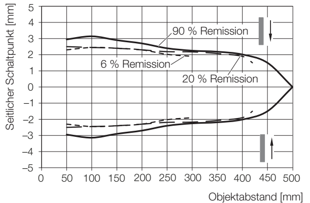
Bild 9-5: Seitlicher Schaltpunkt (...-LH11-...)
