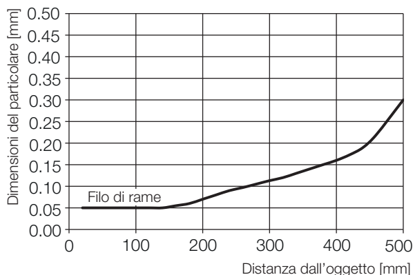
Fig. 9-11: Minimo particolare riconoscibile (...-LH11-...)
