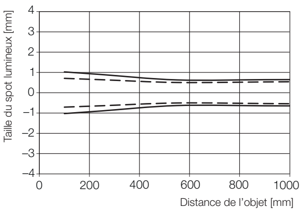
Fig. 9-9: Taille du spot lumineux (...-LH12-...)
