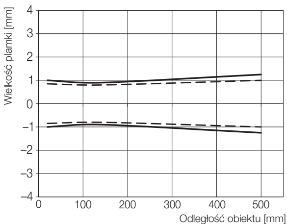
Rys. 9-8: Wielkość plamki światła (...-LH11-...)
