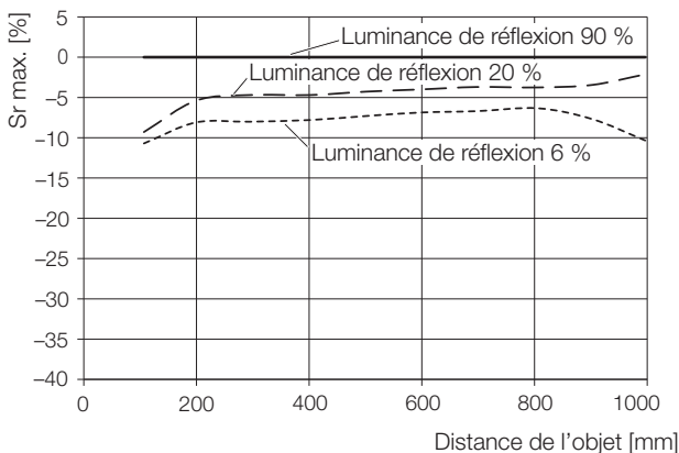
Fig. 9-3: Écart de portée (...-LH12-...)
