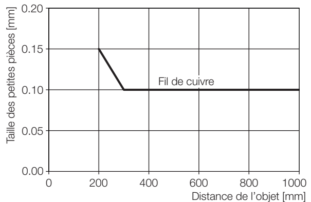
Fig. 9-12: Plus petite pièce reconnaissable (...-LH12-...)
