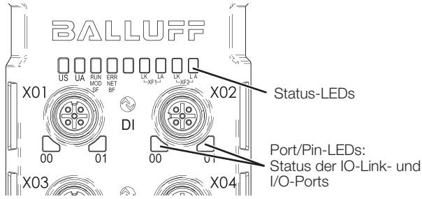
Bild 4-3: Anzeigeelemente
