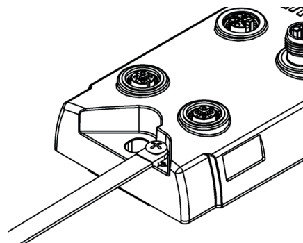
Bild 5-4: Anschluss Erdung
