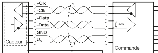
Fig. 2-6 : Exemple de raccordement pour un capteur avec système de commande
