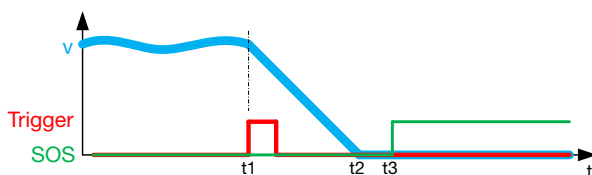
Fig. 2-17: Diagramma corsa-tempo per l'arresto sicuro 2
