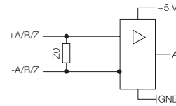
Fig. 2-24 : Circuit de l'électronique consécutive (RS422)
