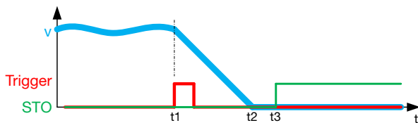
Fig. 2-16: Diagramma corsa-tempo per l'arresto sicuro 1
