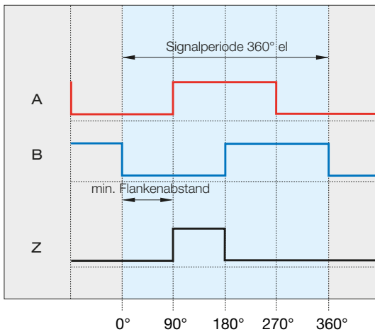
Bild 2-22: Digitale Ausgangssignale bei Vorwärtsbewegung
