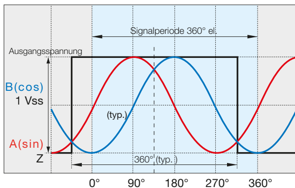
Bild 2-13: Signale des Sinus- und Cosinussensors, Vorwärtsbewegung entspricht ansteigendem Winkel
