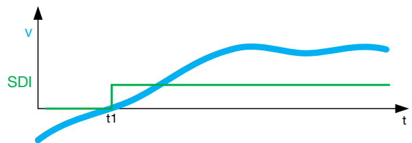
Fig. 2-20: Diagrama de recorrido-tiempo para Sentido del movimiento seguro
