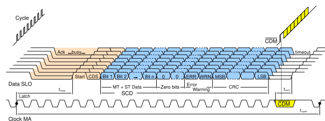
Fig. 2-7: Andamento del segnale interfaccia BiSS-C
