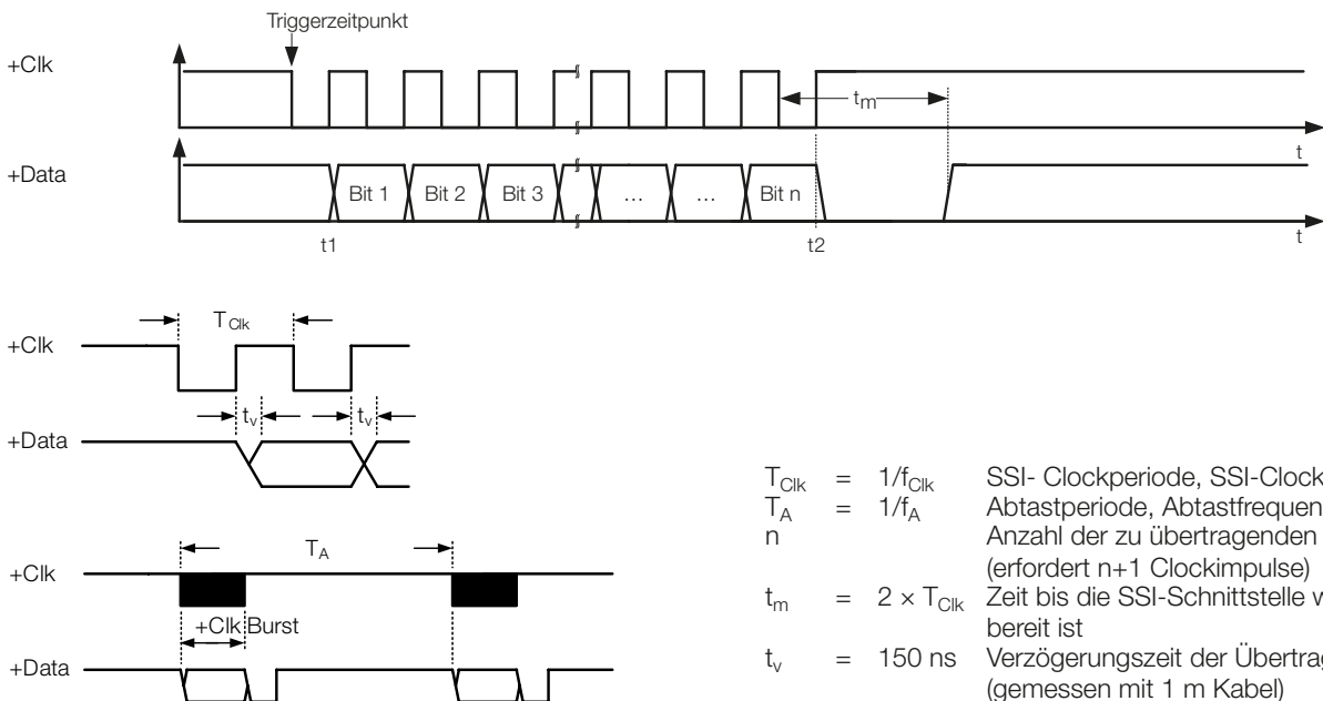
Bild 2-2: Signale bei SSI-Schnittstelle
