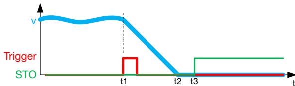
Fig. 2-16: Diagrama de recorrido-tiempo para Parada segura 1
