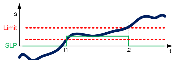
Fig. 2-21 : Diagramme déplacement-temps pour la position limitée sûre
