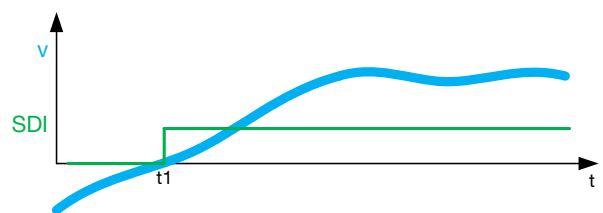
Bild 2-20: Weg-Zeit-Diagramm für Sichere Bewegungsrichtung
