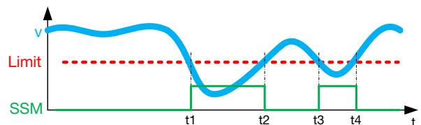
Fig. 2-19: Diagramma corsa-tempo per il monitoraggio della velocità in modo sicuro
