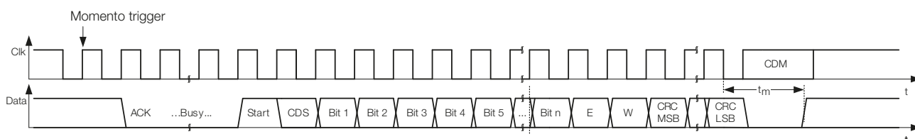
Fig. 2-8: Segnali interfaccia BiSS-C (unidirezionale)
