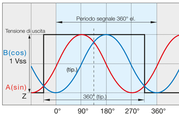
Fig. 2-13: Segnali del sensore sinusoidale e cosinusoidale, il movimento in avanti corrisponde all'angolo crescente
