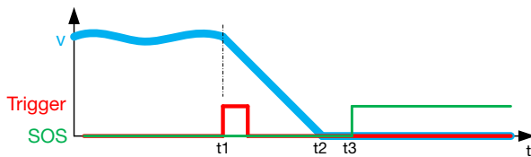
Fig. 2-17: Diagrama de recorrido-tiempo para Parada segura 2
