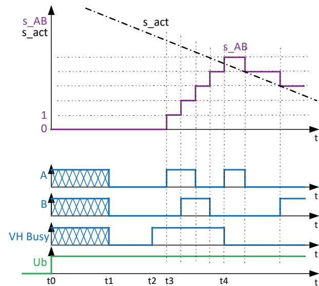
Bild 2-12: Betriebsart "VHBusy"
