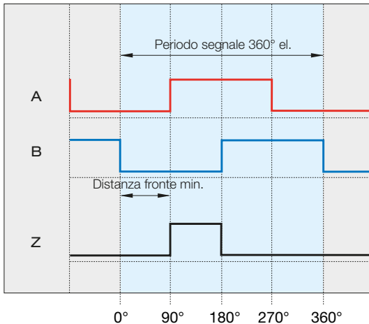
Fig. 2-22: Segnali di uscita digitali nel movimento in avanti
