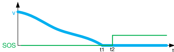
Bild 2-15: Weg-Zeit-Diagramm für Sicherer Betriebshalt
