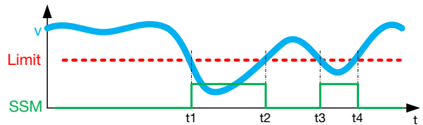
Fig. 2-19: Diagrama de recorrido-tiempo para Monitorización de seguridad segura
