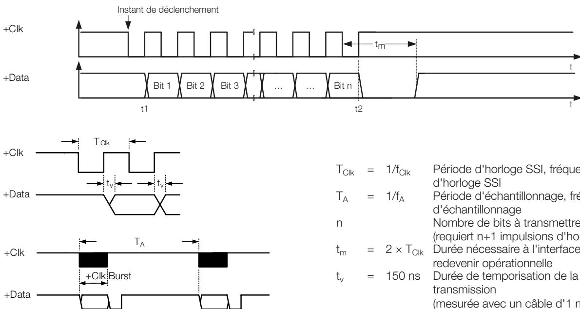
Fig. 2-2 : Signaux pour interface SSI
