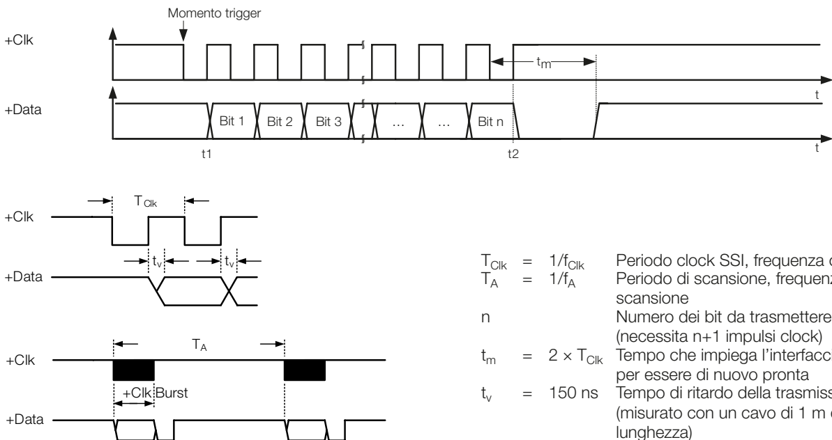
Fig. 2-2: Segnali dell'interfaccia SSI
