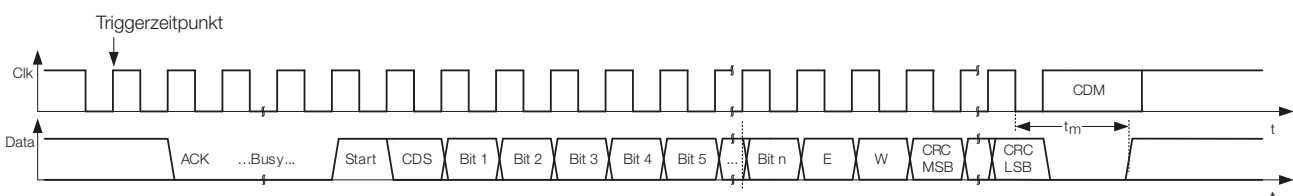
Bild 2-8: Signale BiSS-C-Schnittstelle (unidirektional)
