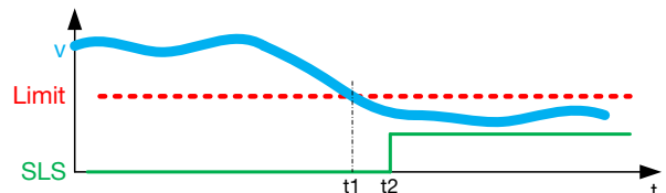
Fig. 2-18: Diagramma corsa-tempo per la Velocità limitata in modo sicuro
