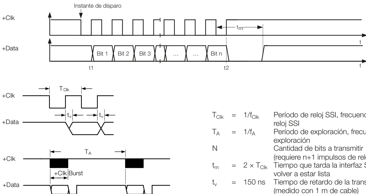
Fig. 2-2: Señales con la interfaz SSI
