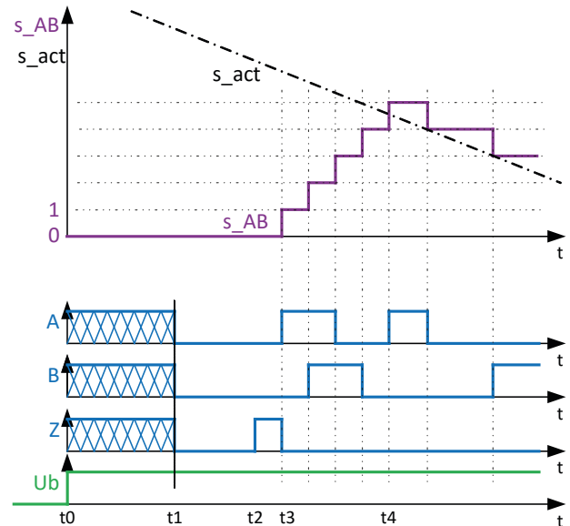
Fig. 2-10: Comportamiento de conexión
