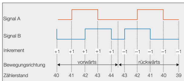
Bild 2-23: Ausgangssignale BML mit Periodenzähler
