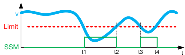
Fig. 2-19 : Diagramme déplacement-temps pour la surveillance de vitesse sûre
