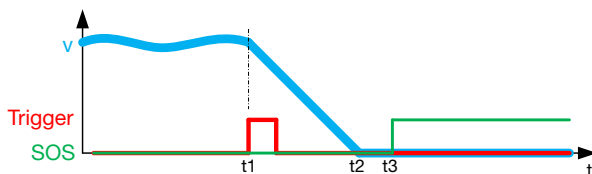
Bild 2-17: Weg-Zeit-Diagramm für Sicherer Stopp 2
