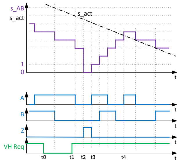
Fig. 2-11: Uso de la entrada VH_{Req}
