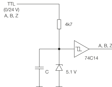
Fig. 2-25 : Circuit de l'électronique consécutive (HTL)
