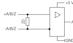
Fig. 2-24: Collegamento elettronica a sequenza (RS422)
