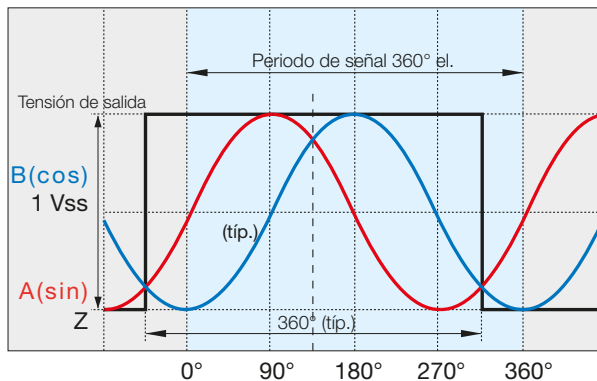
Fig. 2-13: Señales del sensor seno y coseno, un movimiento de avance corresponde a un ángulo ascendente.
