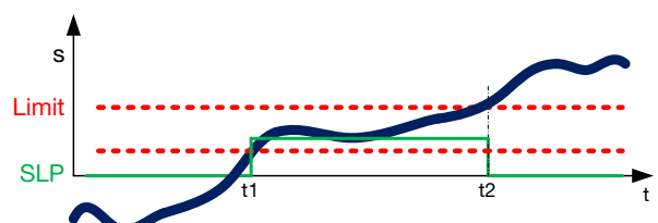
Fig. 2-21: Diagramma corsa-tempo per la Posizione limitata in modo sicuro
