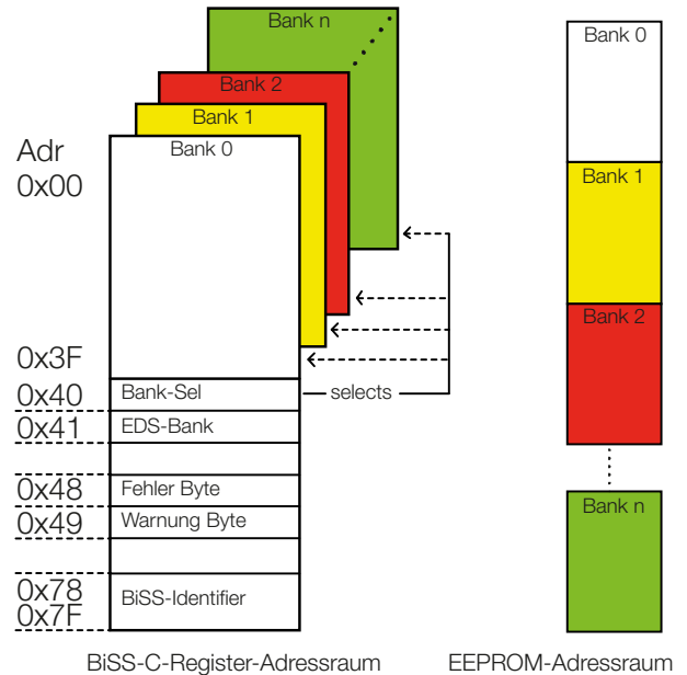
Bild 2-9: BiSS-C-Register-Adressraum
