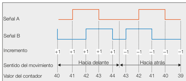
Fig. 2-23: Señales de salida BML con contador de períodos
