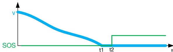
Fig. 2-15 : Diagramme déplacement-temps pour l'arrêt de service de sécurité
