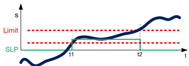
Fig. 2-21: Diagrama de recorrido-tiempo para Posición limitada con seguridad
