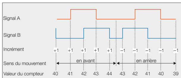
Fig. 2-23 : Signaux de sortie BML avec compteur de périodes
