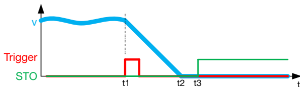
Fig. 2-16 : Diagramme déplacement-temps pour l'arrêt de sécurité 1
