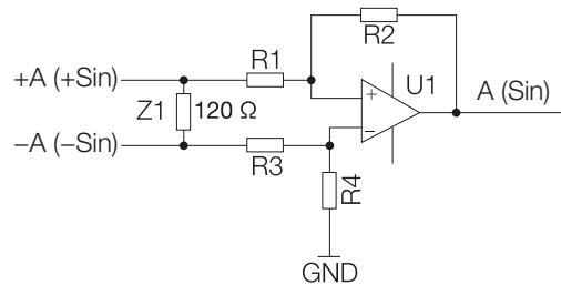
Bild 2-14: Schaltungsbeispiel Folgeelektronik bei Analogausgang +A (+\sin) - (-A (-\sin))
