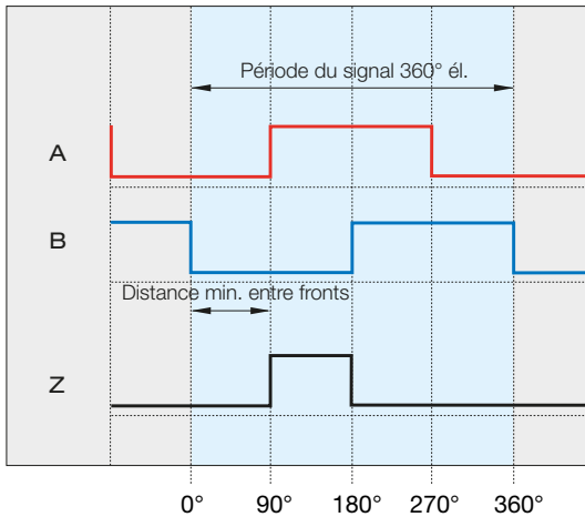
Fig. 2-22 : Signaux de sortie numériques lors du déplacement vers l'avant
