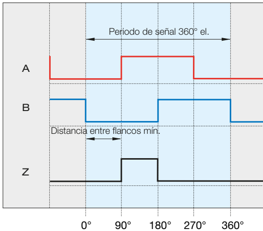
Fig. 2-22: Señales de salida digitales con un movimiento de avance
