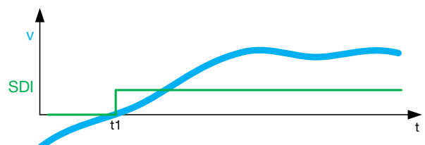
Fig. 2-20: Diagramma corsa-tempo per la direzione di movimento sicura
