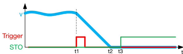
Bild 2-16: Weg-Zeit-Diagramm für Sicherer Stopp 1
