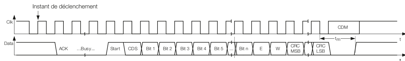
Fig. 2-8 : Signaux de l'interface BiSS C (unidirectionnelle)
