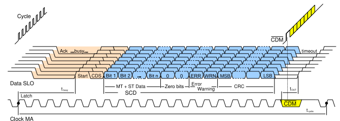
Fig. 2-7: Evolución de la señal con la interfaz BiSS C
