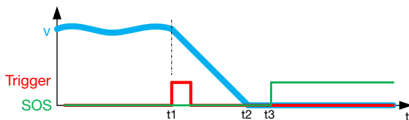
Fig. 2-17 : Diagramme déplacement-temps pour l'arrêt de sécurité 2
