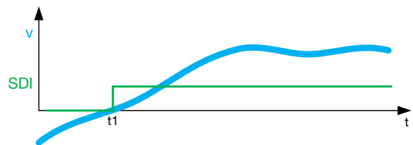
Fig. 2-20 : Diagramme déplacement-temps pour le sens de mouvement sûr
