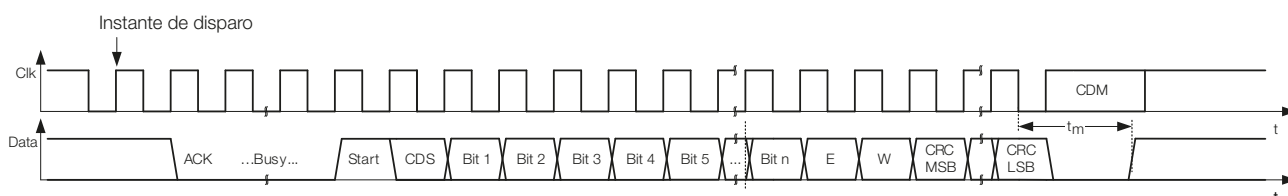
Fig. 2-8: Señales con la interfaz BiSS C (unidireccional)
