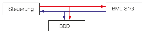
Bild 2-5: Einsatz als Slave
