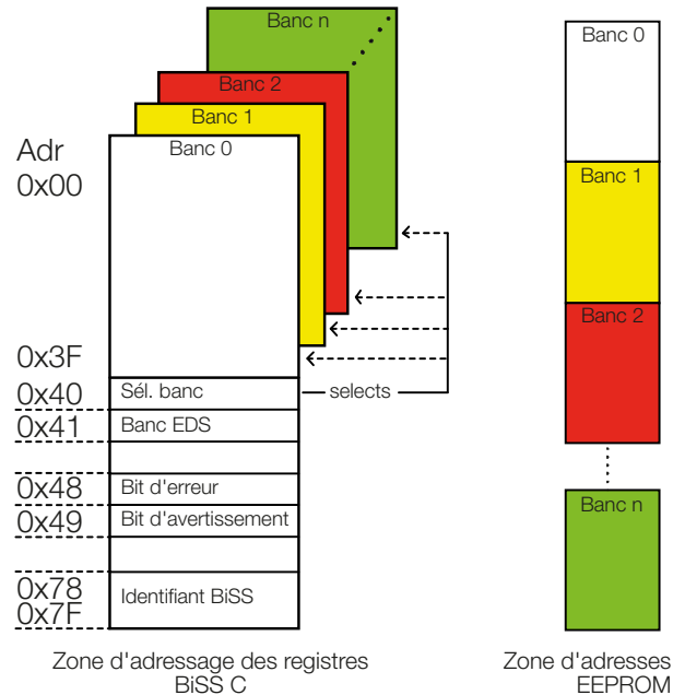
Fig. 2-9 : Zone d'adressage des registres BiSS C
