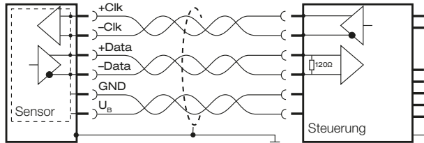
Bild 2-6: Anschlussbeispiel für einen Sensor mit Steuerung
