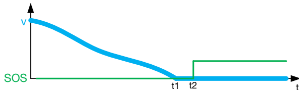
Fig. 2-15: Diagrama de recorrido-tiempo para Parada de servicio segura
