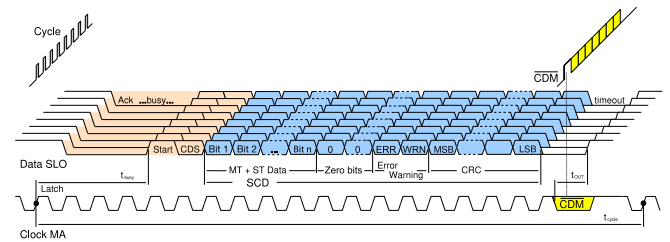
Bild 2-7: Signalverlauf BiSS-C-Schnittstelle
