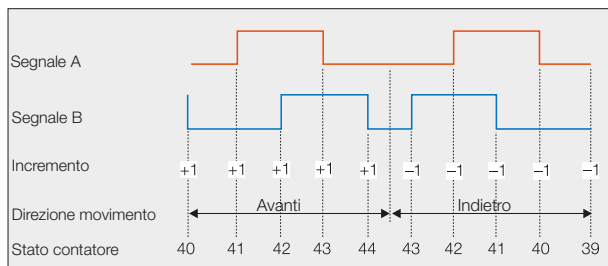
Fig. 2-23: Segnali di uscita BML con contaperiodi
