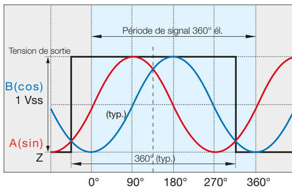
Fig. 2-13 : Signaux du capteur sinus et cosinus ; le déplacement vers l'avant correspond à un angle croissant
