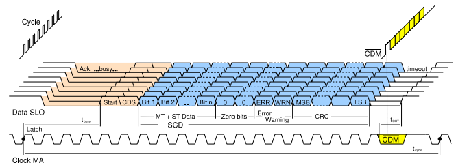
Fig. 2-7 : Parcours du signal de l'interface BiSS C
