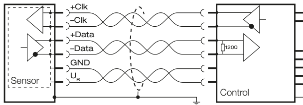
Fig. 2-6: Ejemplo de conexión para un sensor con control
