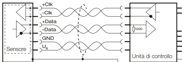
Fig. 2-6: Esempio di collegamento per un sensore con unità di controllo
