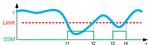
Bild 2-19: Weg-Zeit-Diagramm für Sichere Geschwindigkeitsüberwachung
