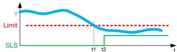
Fig. 2-18 : Diagramme déplacement-temps pour la vitesse limitée sûre
