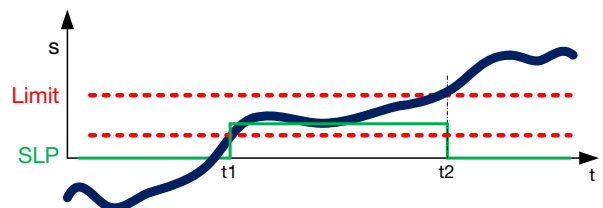
Bild 2-21: Weg-Zeit-Diagramm für Sicher begrenzte Position
