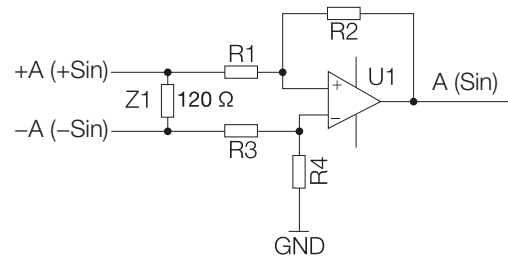
Fig. 2-14: Esempio di circuito elettronico a sequenza nell'uscita analogica +A (+sin) - (-A (-sin))
