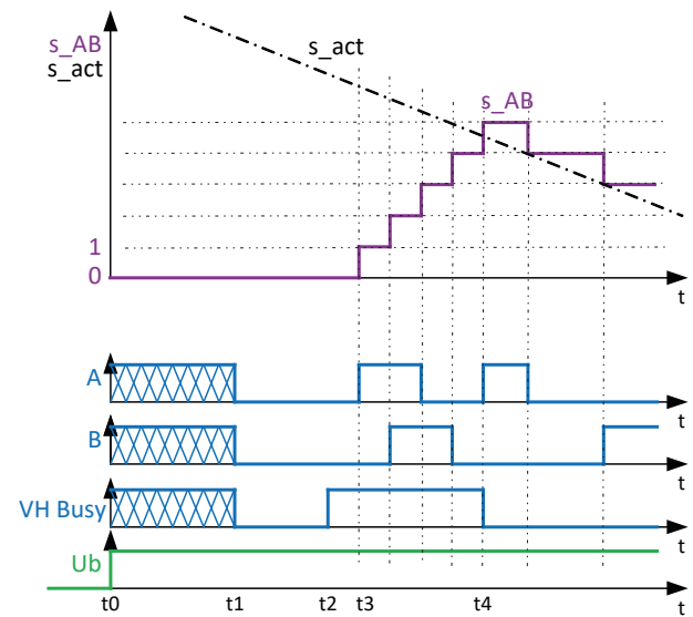
Fig. 2-12 : Mode « VHBusy »
