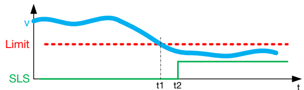
Fig. 2-18: Diagrama de recorrido-tiempo para Velocidad limitada con seguridad
