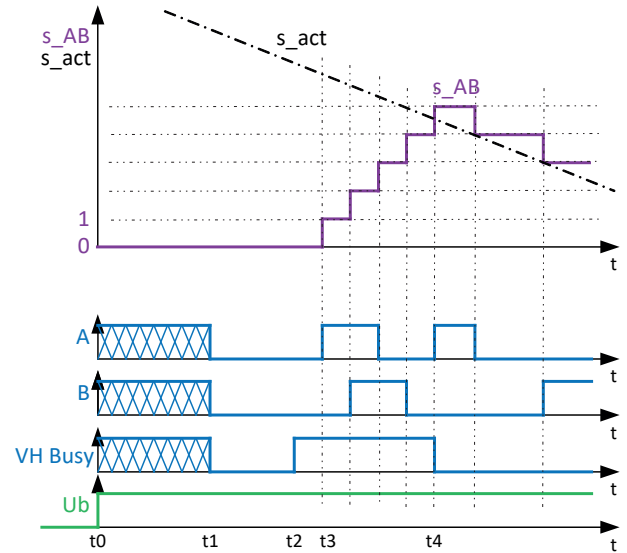
图 2-11: “VH Busy” 模式
