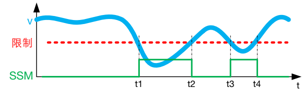
图 2-22: 安全转速监控的距离-时间图
