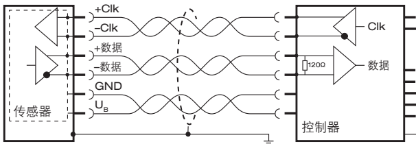
图 2-5: 传感器与控制器接线样例
