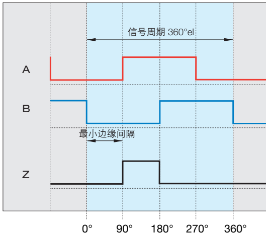
图 2-25: 向前移动的数字量输出信号
