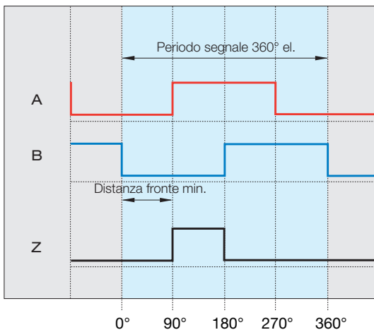
Fig. 2-25: Segnali di uscita digitali nel movimento in avanti
