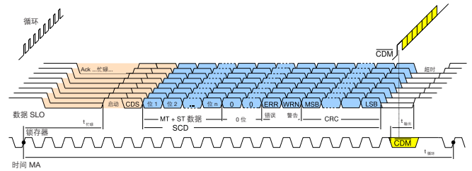
图 2-6: BiSS C 接口的信号序列
