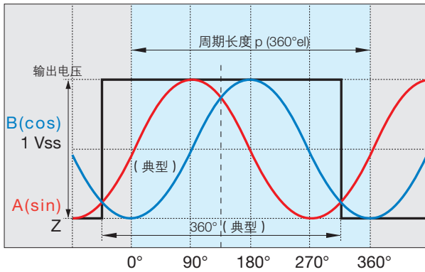
图 2-12: 对于 sin/cos 接口 (1Vpp) 的信号，正向运动对应于增加角度
