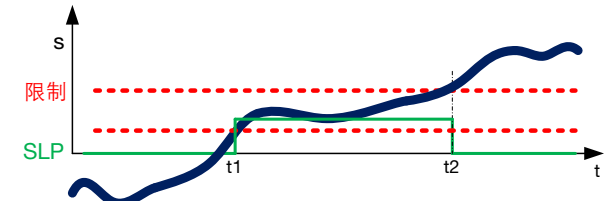
图 2-24: 安全限制位置的行程-时间图
