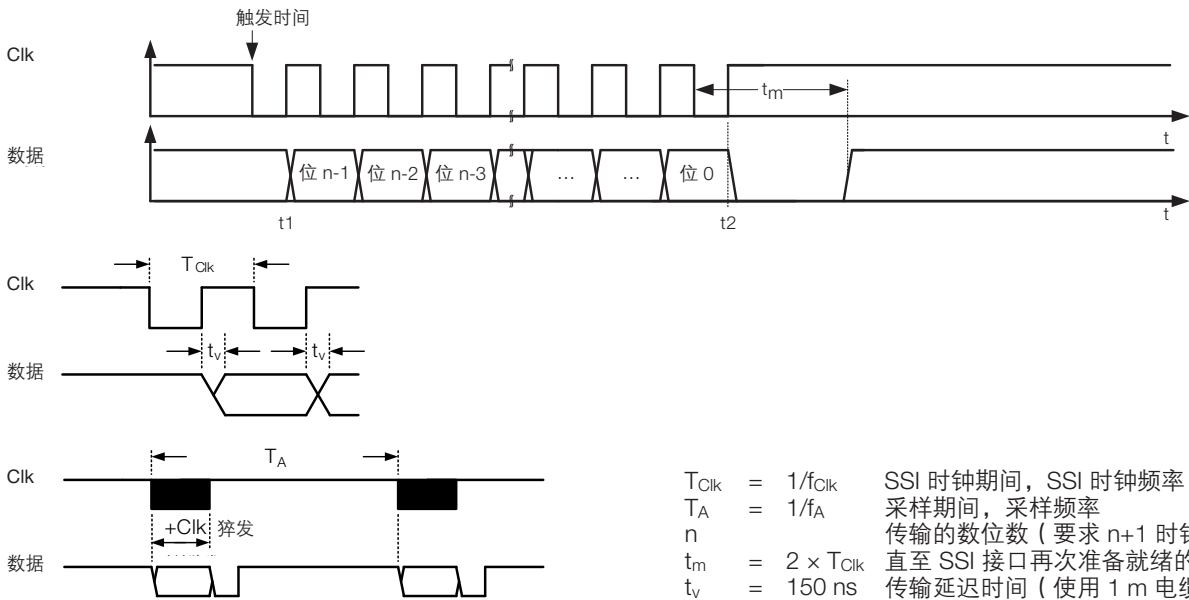
图 2-2: SSI 接口的信号
