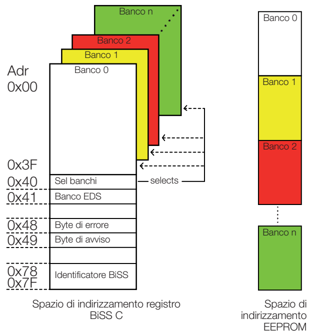
Fig. 2-8: Spazio di indirizzamento registro BiSS C
