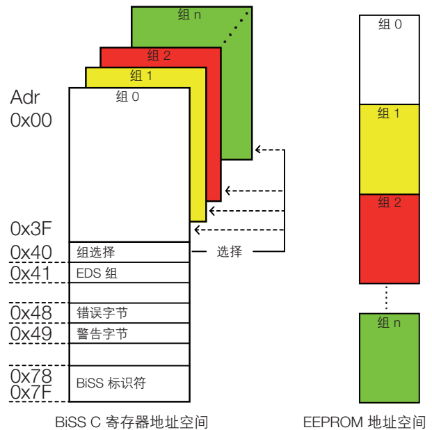
图 2-8: BiSS C 寄存器地址空间
