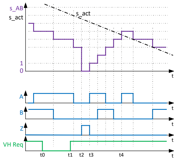
图 2-10: 使用输入 VH_{Req}
