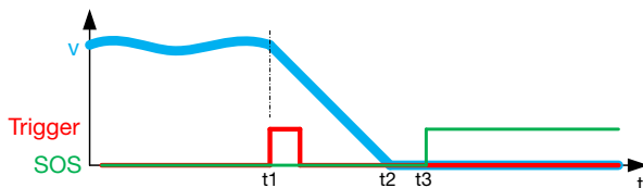
Fig. 2-20: Diagrama de recorrido-tiempo para Parada segura 2
