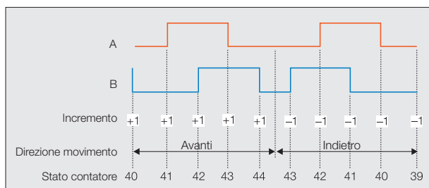
Fig. 2-26: Segnali di uscita BML con contaperiodi per analisi quadrupla nell'unità di controllo
