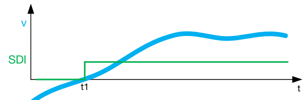
图 2-23: 安全方向的距离-时间图
