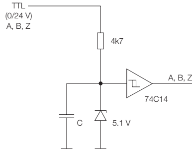
图 2-28: 高阈值逻辑电路 (HTL)
