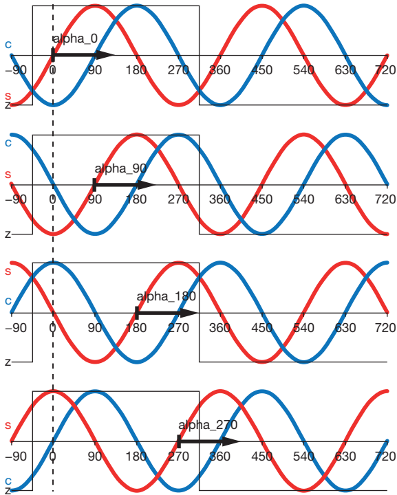
图 2-15: s、c 和 z 的四种不同相位关系
