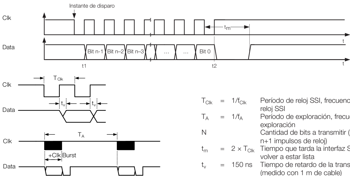
Fig. 2-2: Señales con la interfaz SSI
