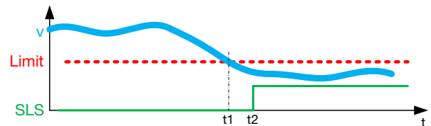
Fig. 2-21: Diagrama de recorrido-tiempo para Velocidad limitada con seguridad
