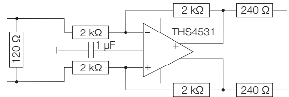
图 2-13: 一个通道有一个差值运算放大器的滤波电路。
