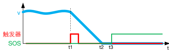
图 2-20: 安全停止 2 的距离-时间图
