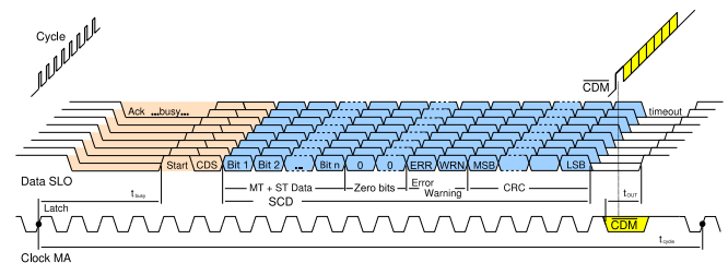
Bild 2-6: Signalverlauf BiSS-C-Schnittstelle
