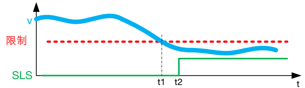
图 2-21: 安全限速的距离-时间图
