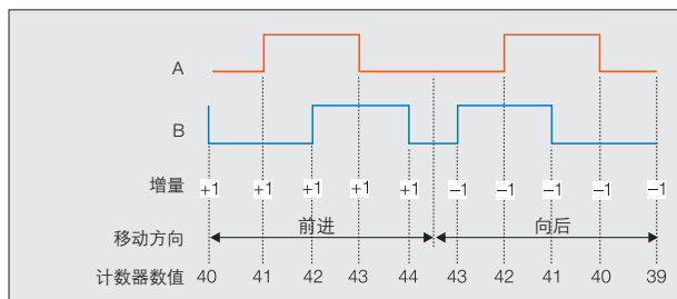
图 2-26: BML 输出通过周期计数器输出信号, 用于控制器中的 4x 插值
