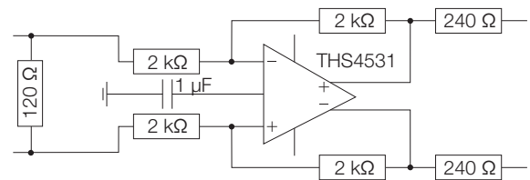
Fig. 2-13: Conmutación de filtro con un amplificador de operación diferencial para un canal.
