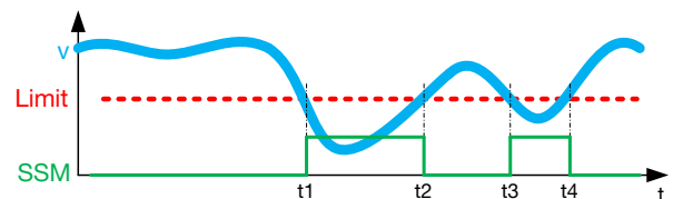
Fig. 2-22: Diagrama de recorrido-tiempo para Monitorización de seguridad segura
