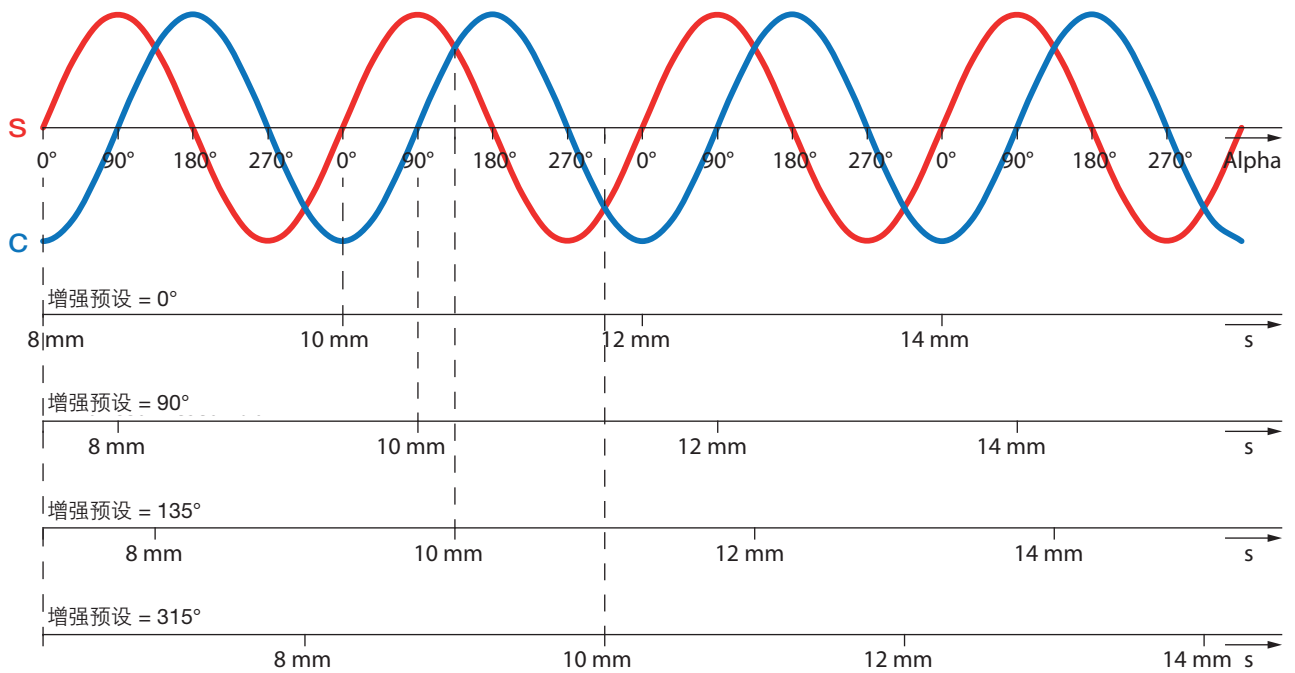
图 2-17: 增强预设不同角度的 sin/cos 信号与绝对位置之间的角度关系
