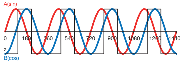
图 2-14: 磁极周期参考点功能信号
