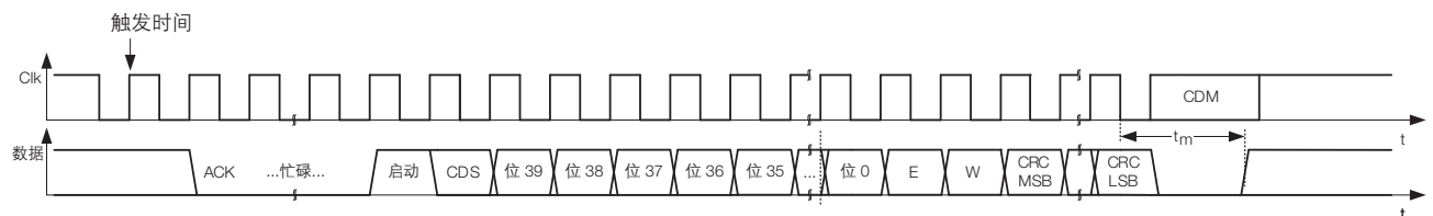
图 2-7: BiSS C 接口信号 (单向)
