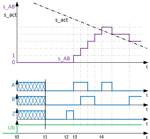
图 2-9: 接通操作
