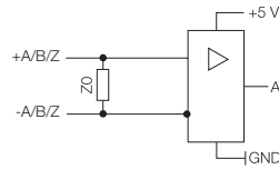
图 2-27: 后续电子电路 (RS422)
