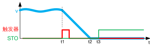
图 2-19: 安全停止 1 的距离-时间图
