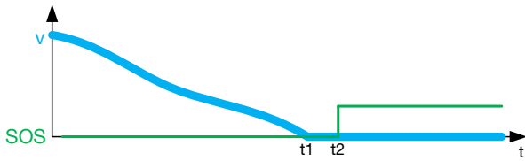
图 2-18: 安全运行停止的距离-时间图
