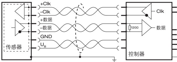
图 2-1: 传感器与控制器接线样例
