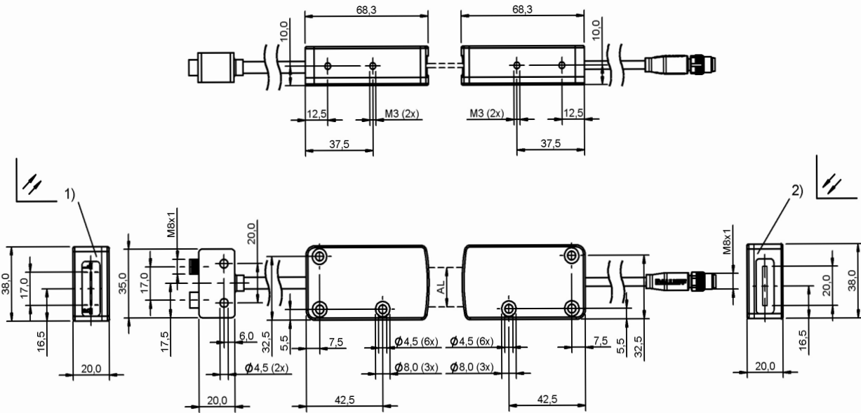
1) Empfänger 2) Sender
