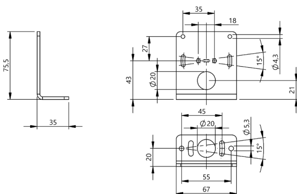
Abbildung 3-1: Maße
