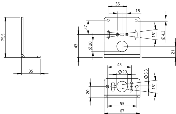
Fig. 3-1: Dimensions
