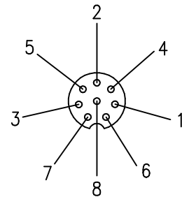
Ansicht auf Anschlußseite der Einsätze
