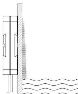
Fig. 5-2 : Étalonnage « vide » avec dépôts adhérents
