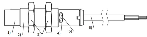
Bild 3-2: Aufbau der Kabelausführung, 1) Aktive Fläche, 2) Befestigungsgewinde M12x1, 3) Befestigungsmuttern, 4) Anzeige Sensorzustand (grüne LED), 5) Anzeige Schaltzustand (gelbe LED), 6) Anschlusskabel
