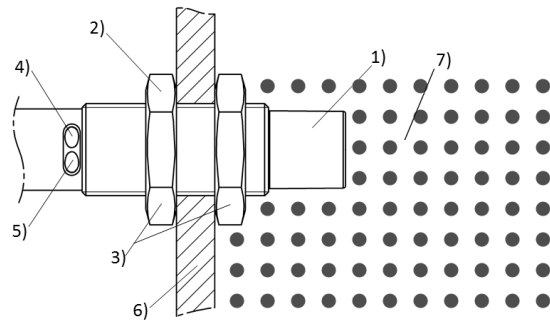
Bild 5-3: Abgleich mit Schüttgut, 1) Aktive Fläche, 2) Befestigungsgewinde M12x1, 3) Befestigungsmutter, 4) Anzeige Sensorzustand (grüne LED), 5) Anzeige Schaltzustand (gelbe LED), 6) Behälterwand, 7) Schüttgut
