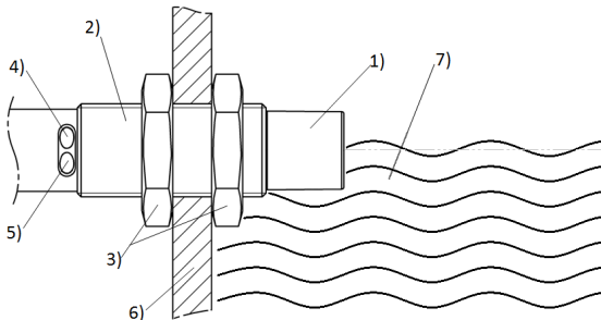
Bild 5-2: Abgleich zur Füllstanderkennung, 1) Aktive Fläche, 2) Befestigungsgewinde M12x1, 3) Befestigungsmutter, 4) Anzeige Sensorzustand (grüne LED), 5) Anzeige Schaltzustand (gelbe LED), 6) Behälterwand, 7) Flüssigkeit
