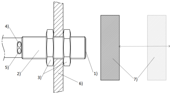
Bild 5-1: Abgleich zur Objekterkennung, 1) Aktive Fläche, 2) Befestigungsgewinde M12x1, 3) Befestigungsmutter, 4) Anzeige Sensorzustand (grüne LED), 5) Anzeige Schaltzustand (gelbe LED), 6) Behälterwand, 7) Objekt
