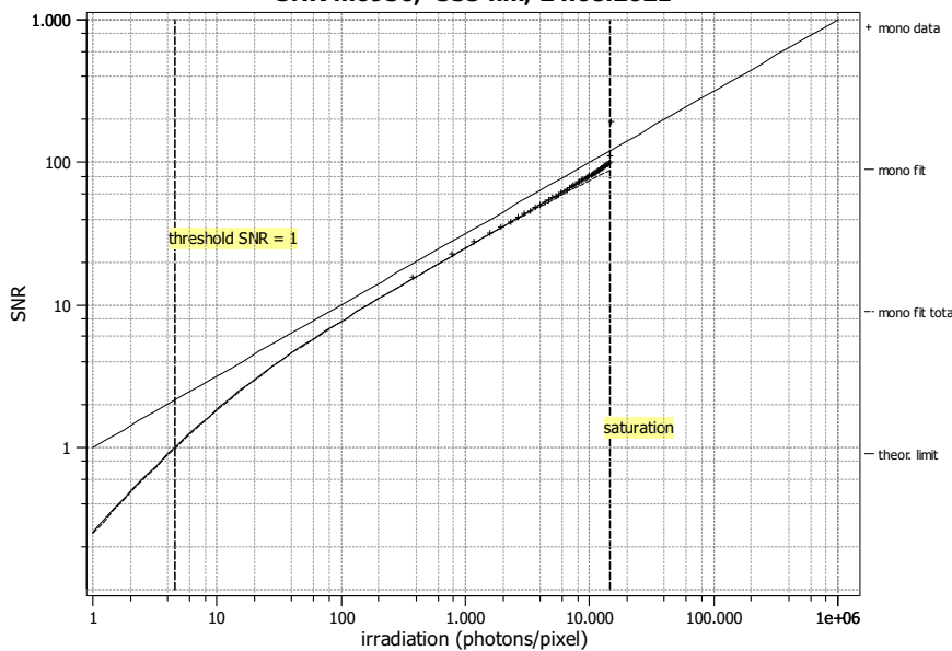
SNR m0950, 535 nm, 24.08.2021
